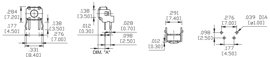
P.C.B LAND PATTERN
